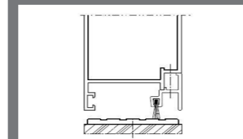
provedení bez prahu (lišta 3 mm + kartáč)
