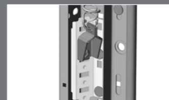
kotvení pružin
